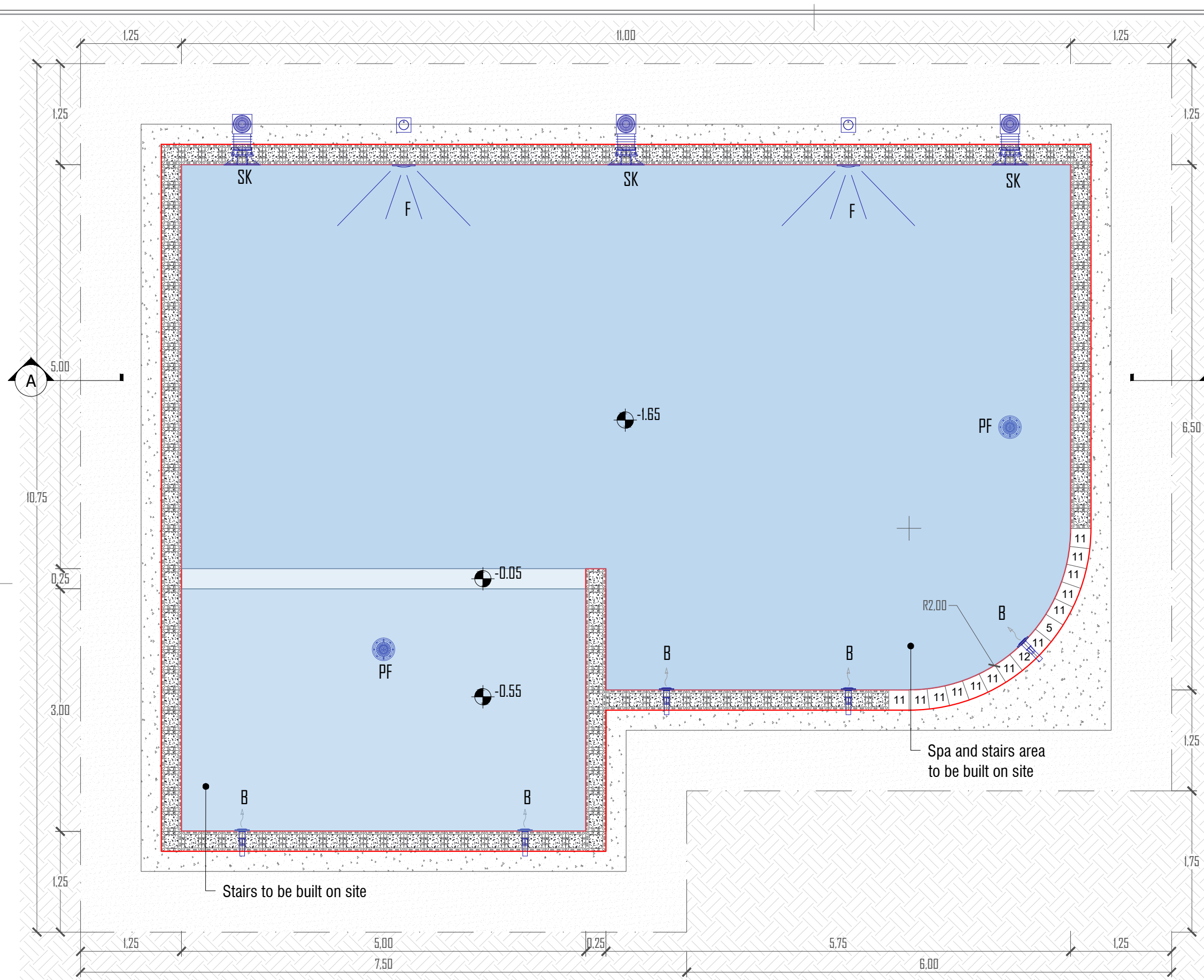
1 PLANIMETRIA GENERALE Sc.: 1:50 0 50cm 100cm
